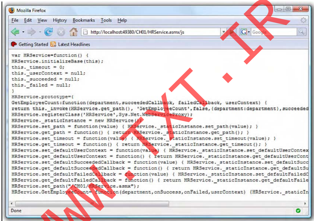
شکل ۱۲-۵ پروکسی جاوااسکریپت برای فرخوانی سرویس وب
